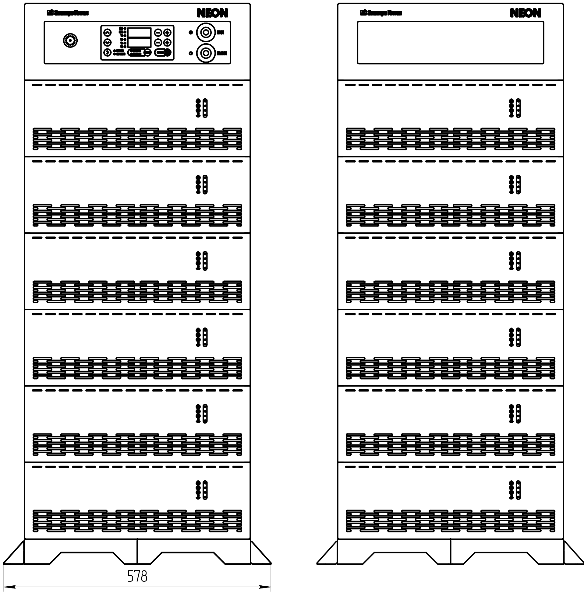
Вид спереди
