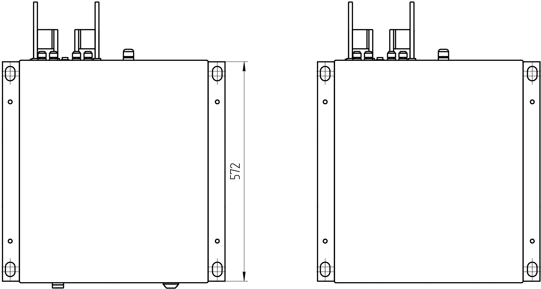
Вид сверху
